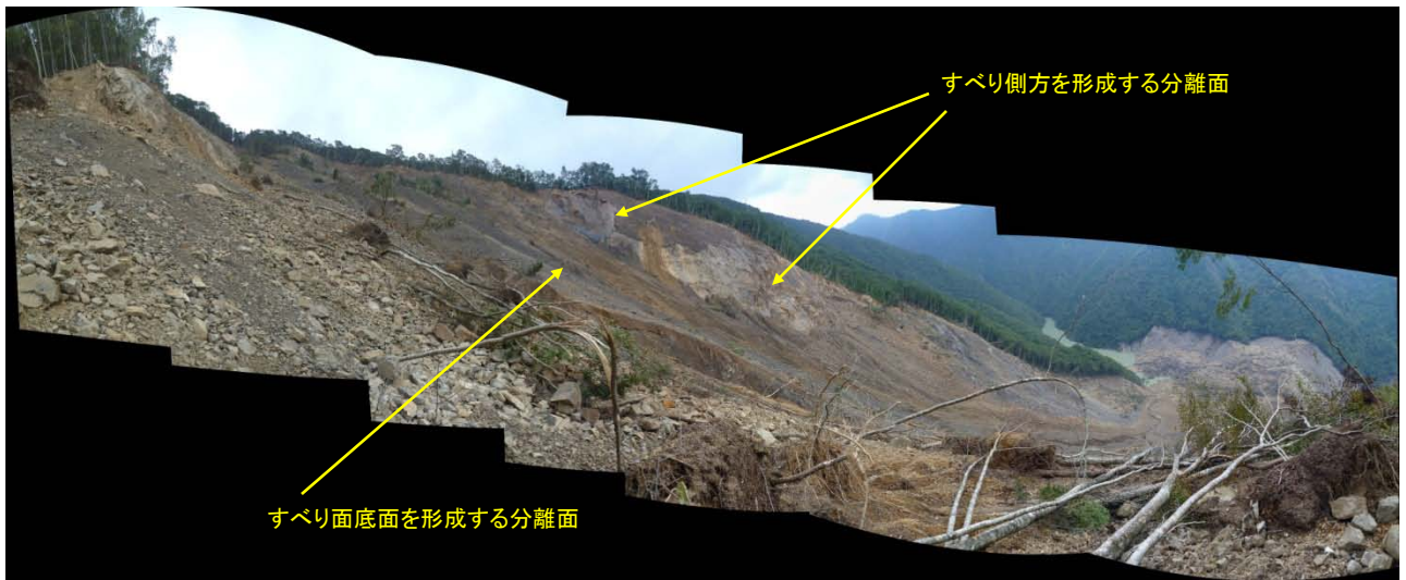
下流標高810m付近から見た崩壊地
